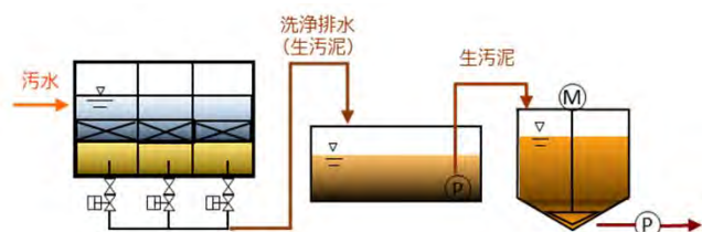
(1) 超高効率固液分離設備 (2) 生汚泥貯留設備 (3) 一次濃縮設備
