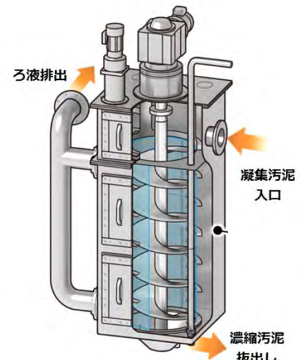
高濃度対応型ろ過濃縮機
