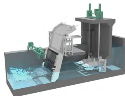
ポンプゲート形(ゲート有り)
