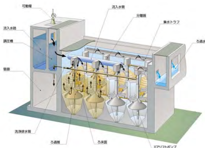
本技術の構造例(大規模向けRC造)
