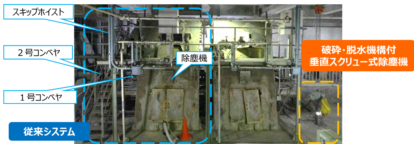
設置状況例(床上部分)
