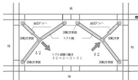
増幅機構付き制震装置による制震補強
