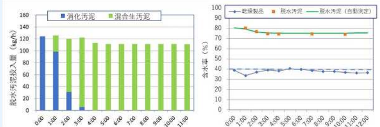
投入汚泥の性状変動の試験 (例)
