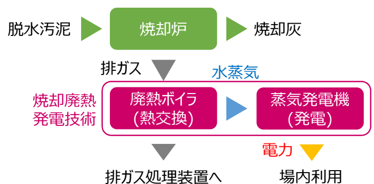
焼却廃熱発電の概念図
