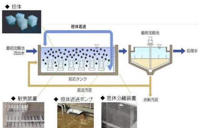
処理水量増加対応型 処理フロー
