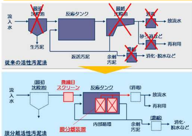
従来の活性汚泥法とMBRの処理フローの比較
