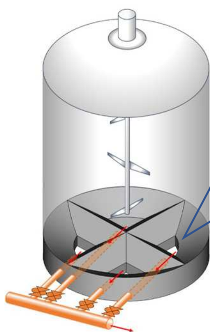
4分割ピット構造
