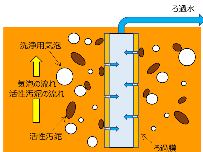
MBRにおける膜ろ過の概念図
