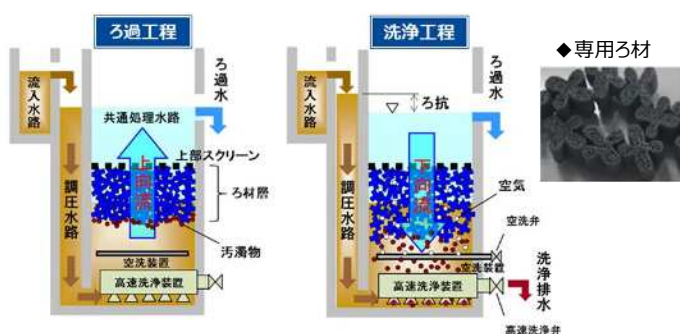
ろ過池の基本原則
