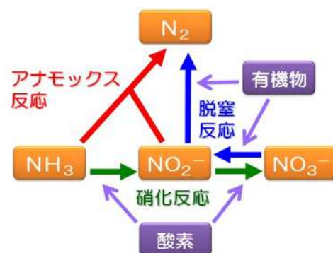
窒素循環の模式図
