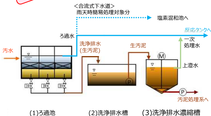
初沈代替高速ろ過システム 処理フロー
