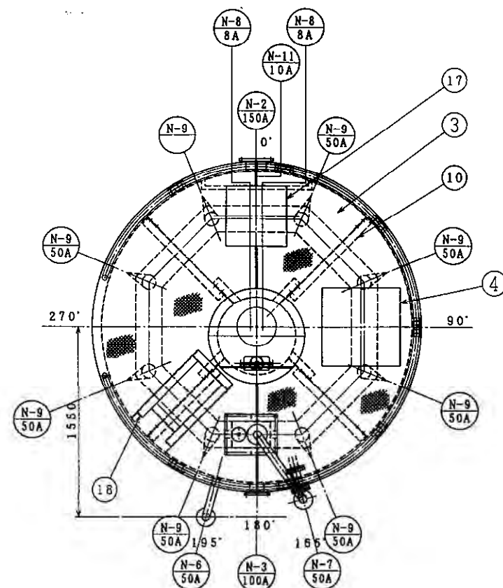
矢視 A~A
