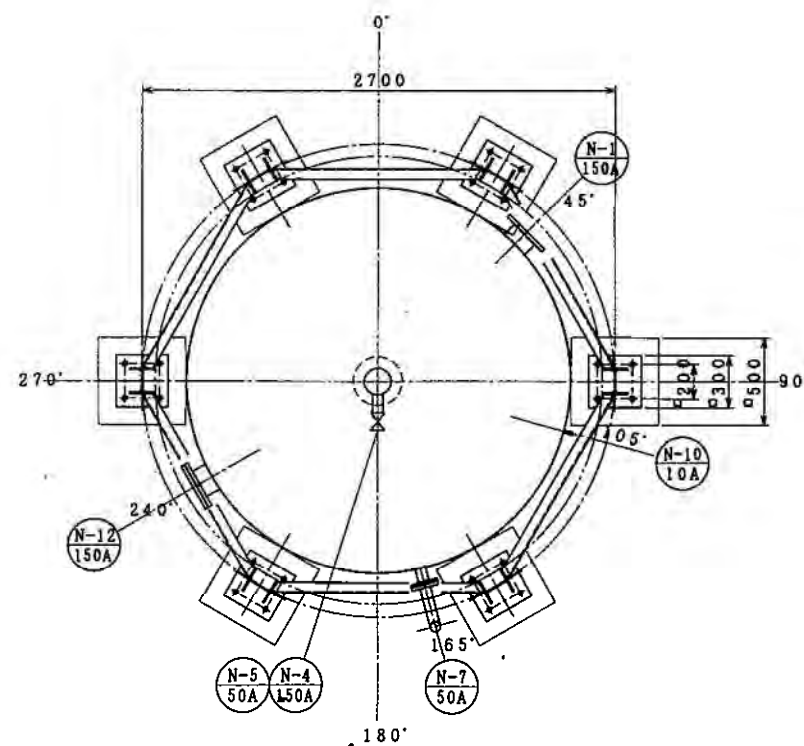
矢視 B~B
