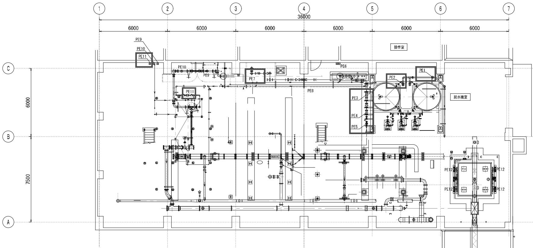
汚泥処理棟2階（下部）平面図 S=1/100
