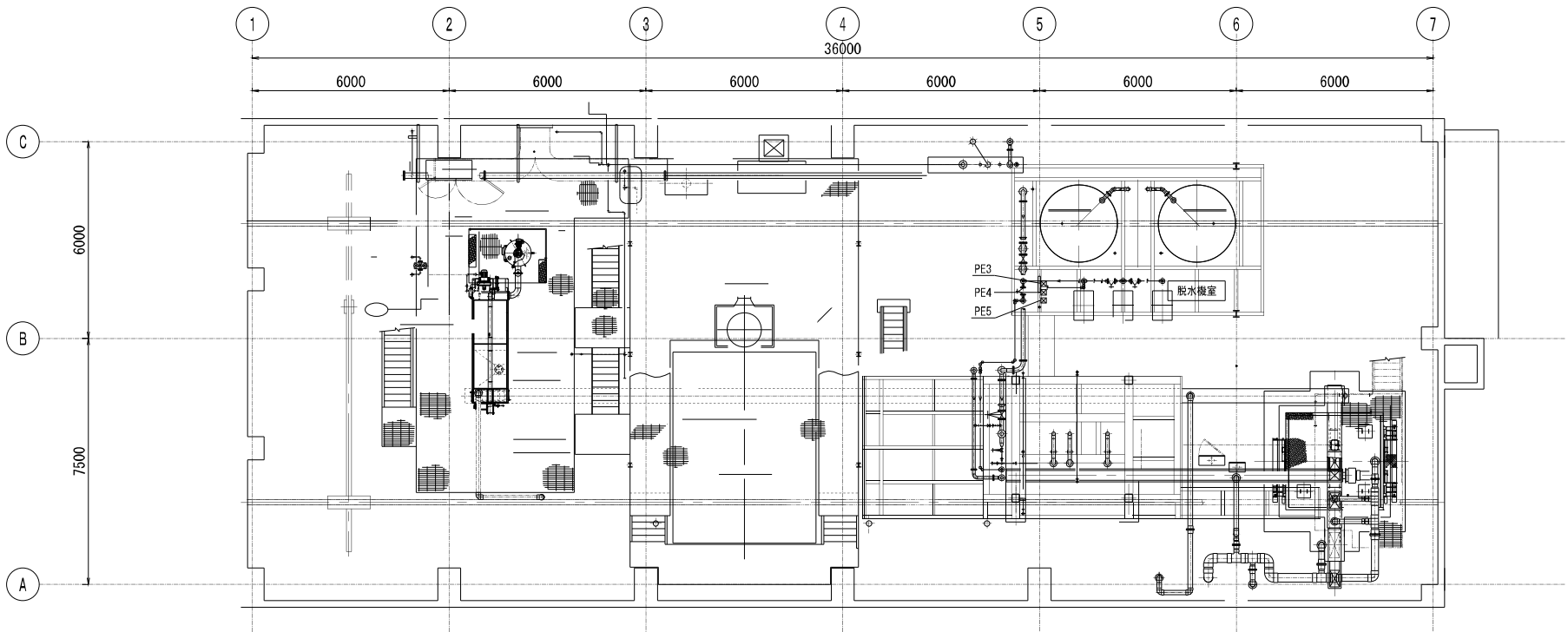
汚泥処理棟2階（上部）平面図 S=1/100
