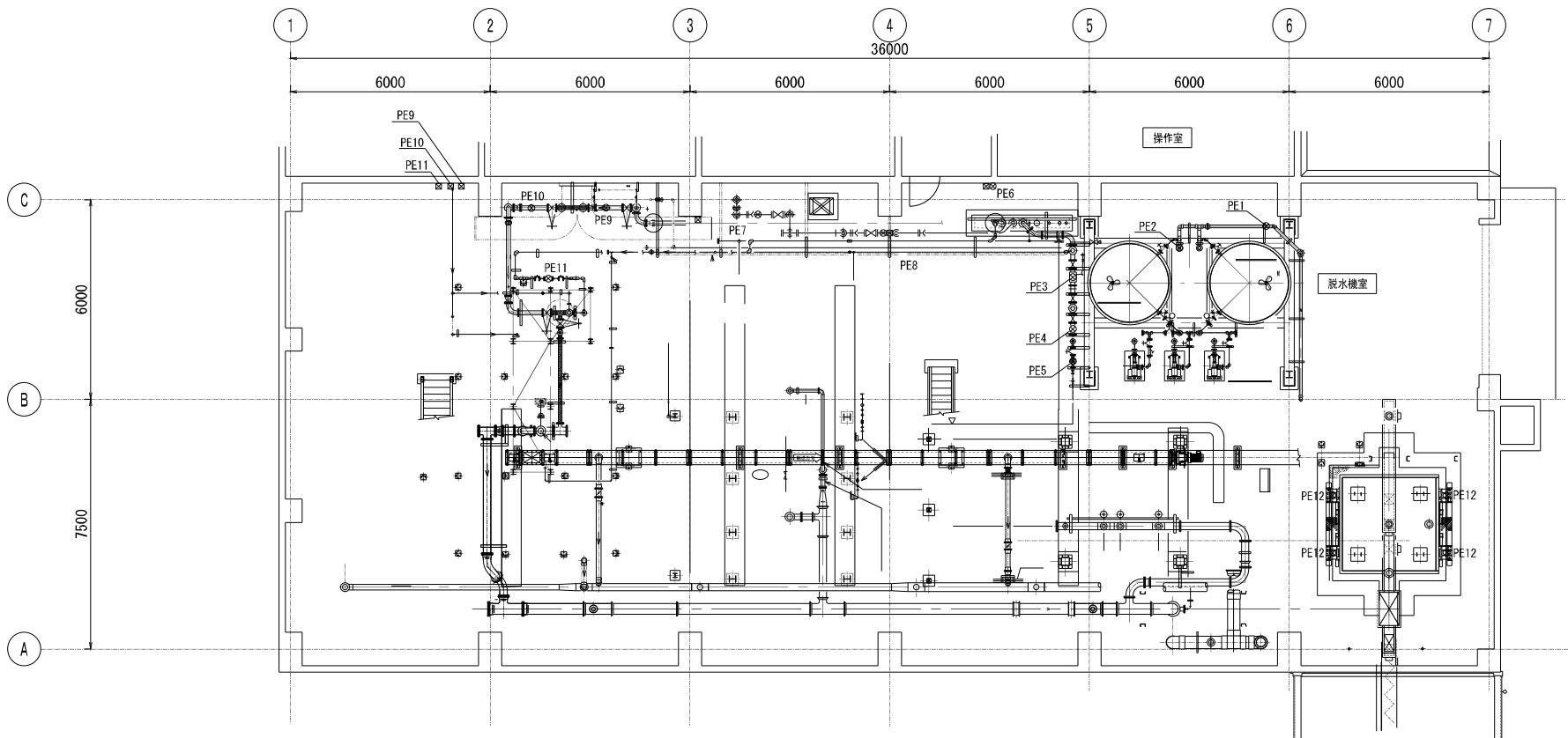
汚泥処理棟2階（下部）平面図 S=1/100
