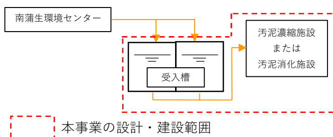
図 2 し尿・浄化槽汚泥受入れ取合区分図
